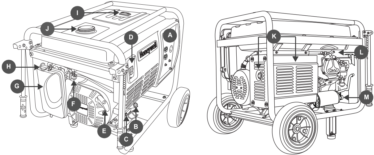
FIGURA 14: Generador portátil HW6200L
