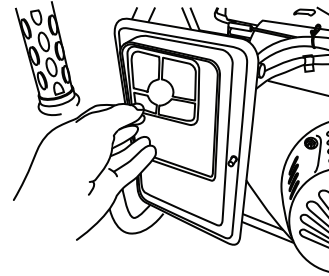
FIGURA 39: Instalación de la placa del filtro de aire - Modelo HW6200
