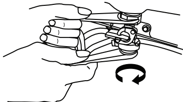
FIGURA 48: Suelte el perno para drenar el combustible
